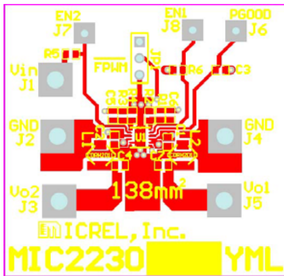
Top Layer
